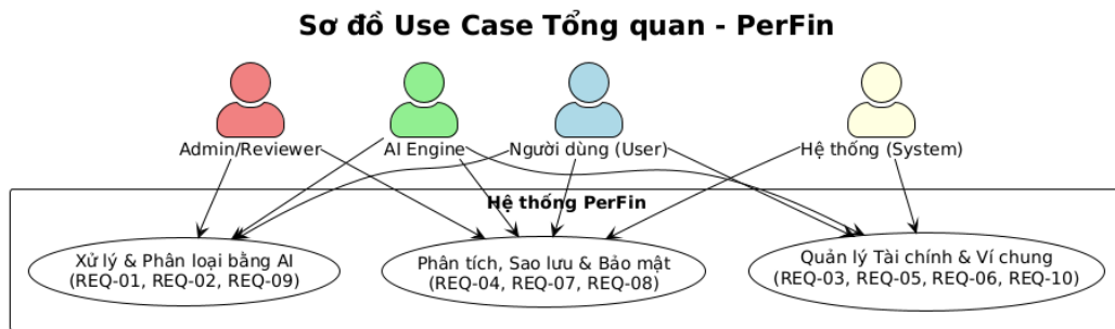
Figure 3.4: Sơ đồ Use Case tổng quan mức cao (Overview)
